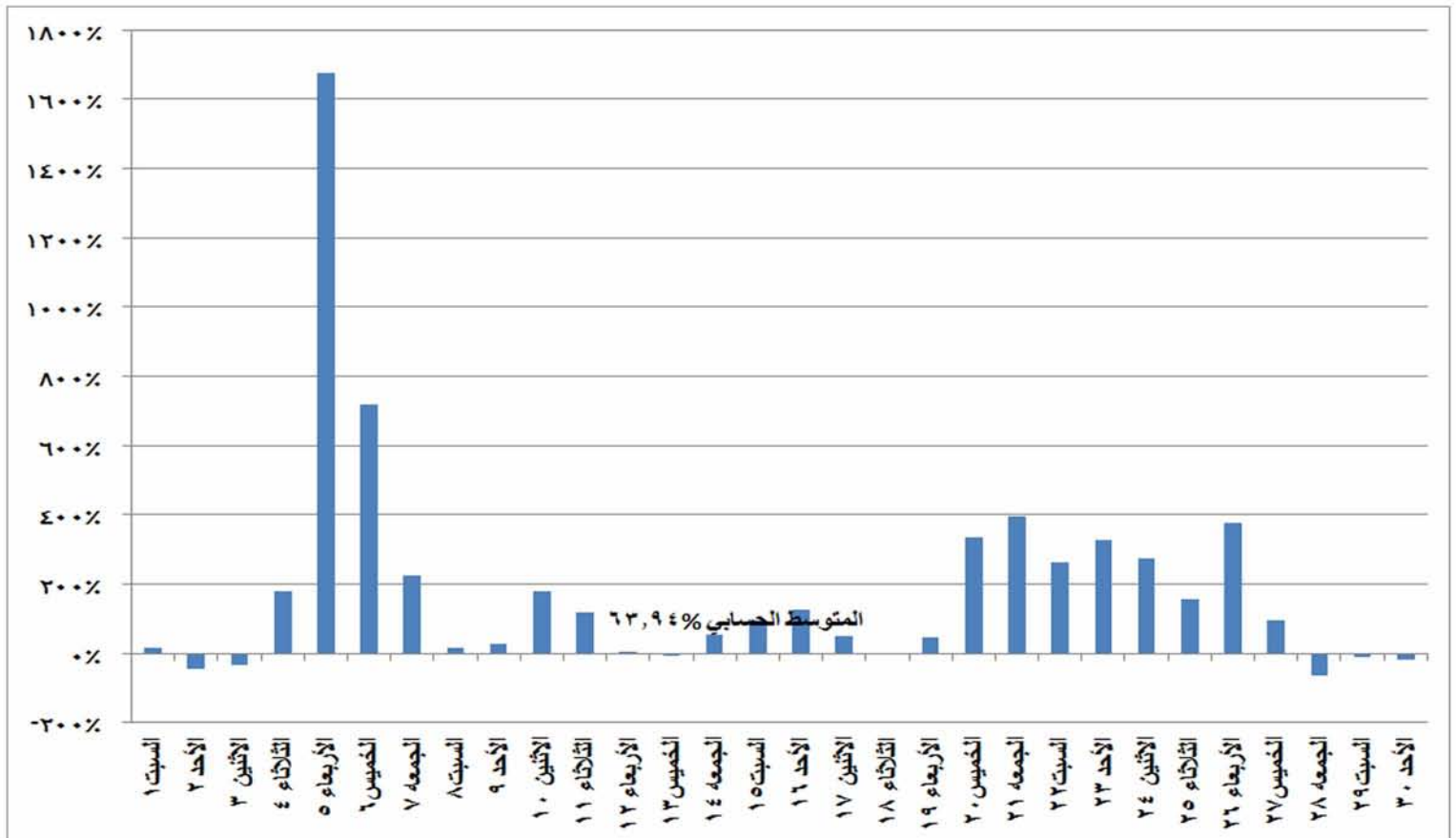
شكل (٢٦) نسب التغير في استخدام الرياح والشمس في إنتاج الطاقة الكهربائية خلال شهر أكتوبر ٢٠١٦ مقارنة بالشهر المماثل من العام السابق
