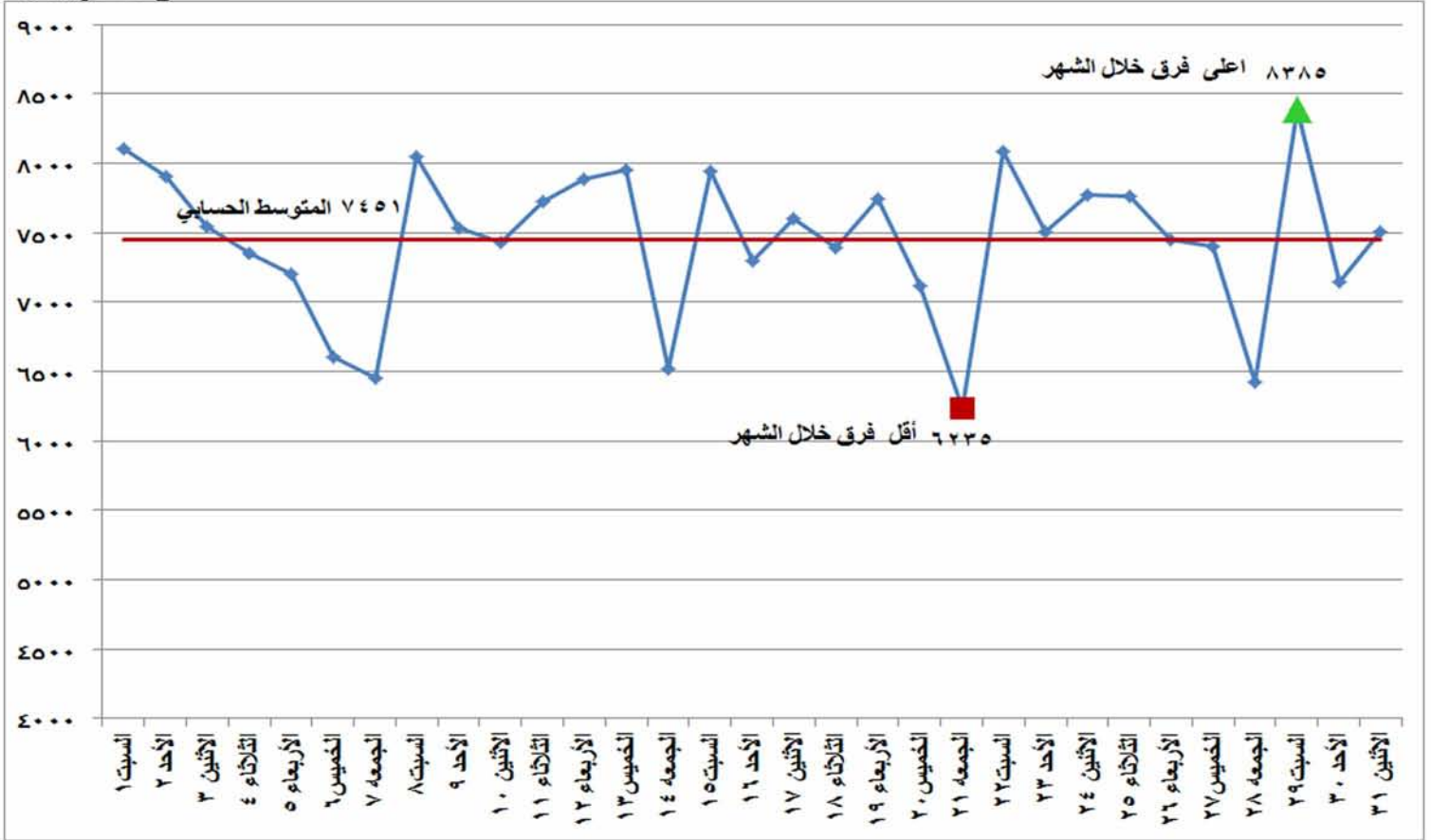
شكل (٣) الفرق بين أقصى وأدنى حمل خلال شهر أكتوبر ٢٠١٦
