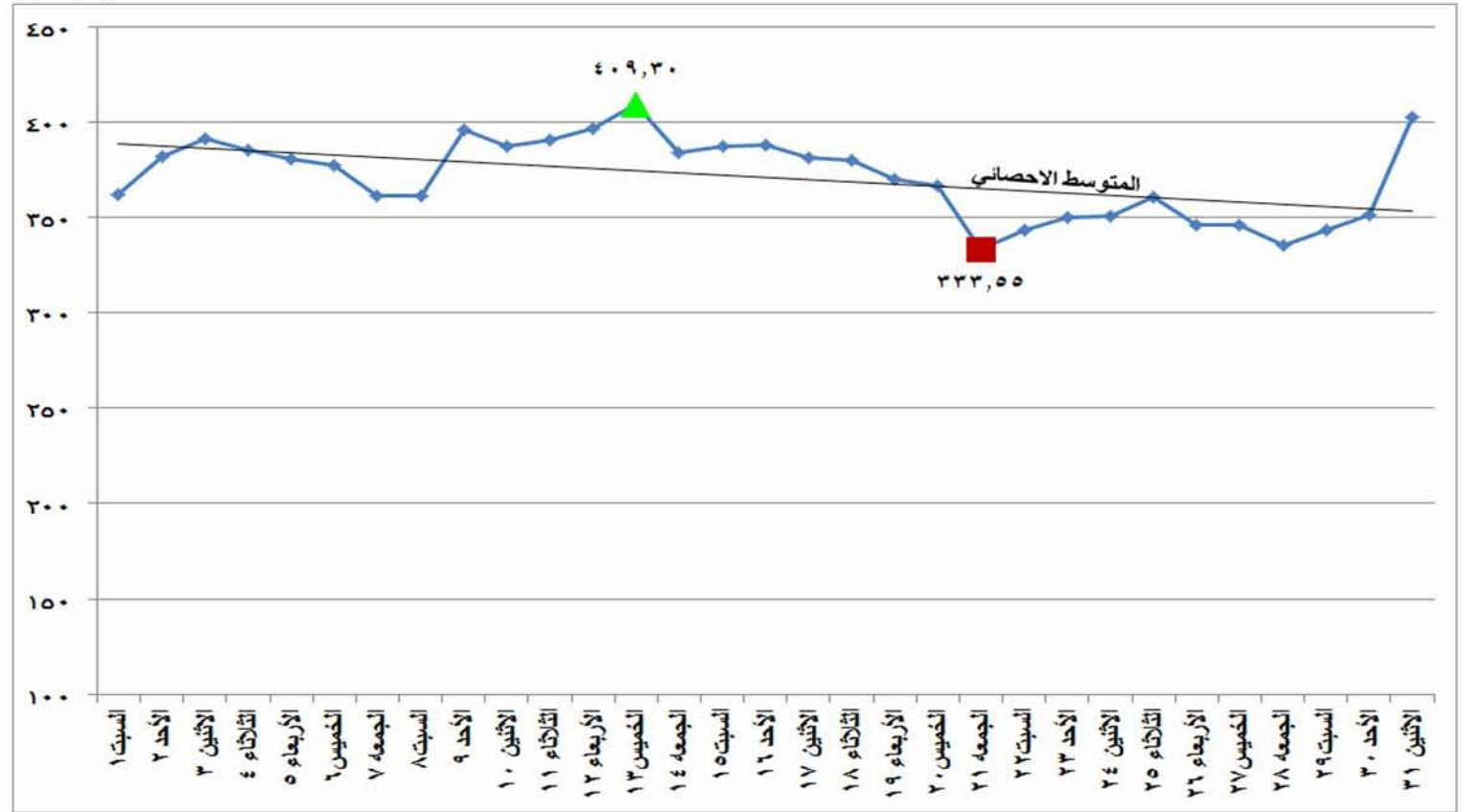
شكل (١٧) الطاقة الكهربائية المنتجة من الغاز الطبيعي خلال شهر أكتوبر ٢٠١٦
