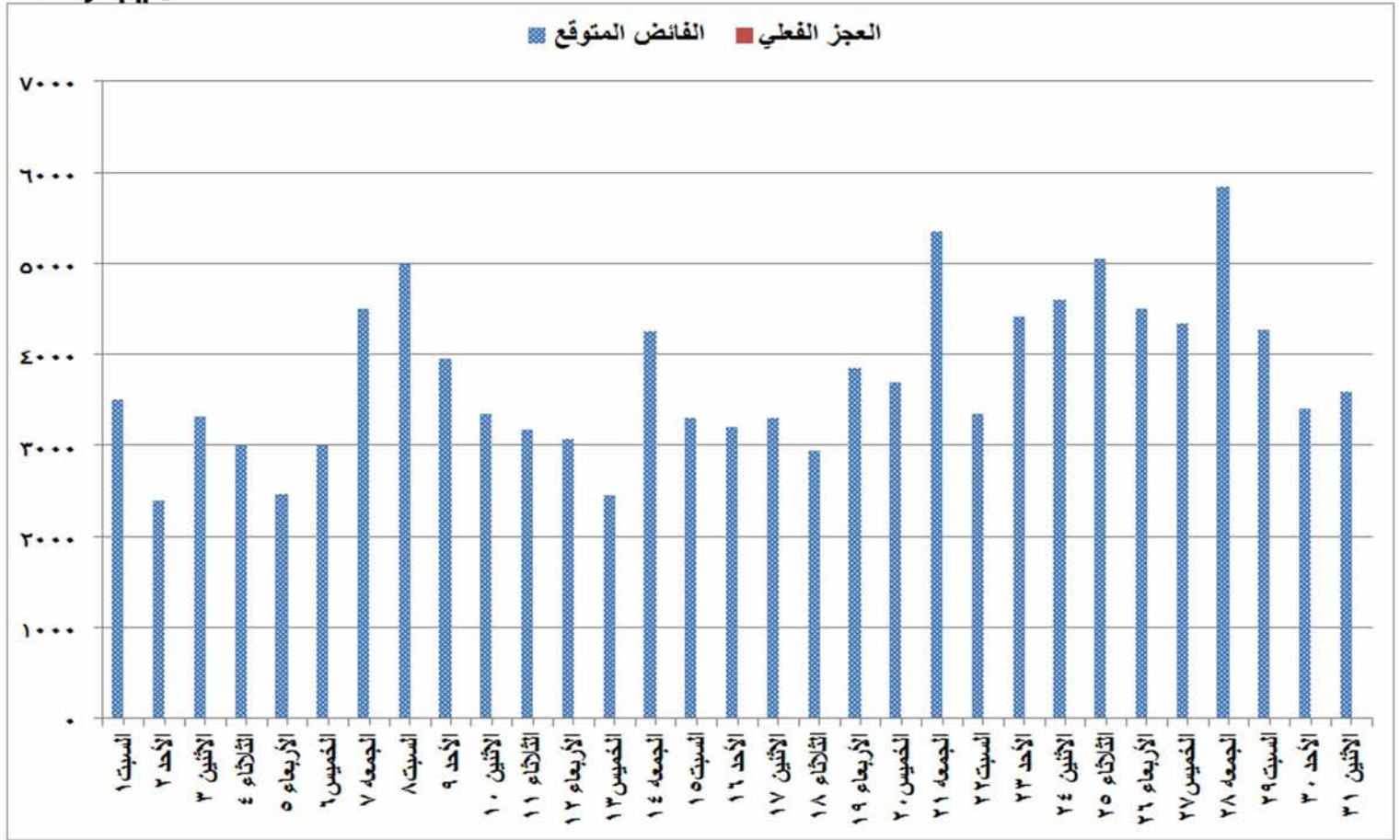
شكل (٧) الفائض والعجز المتوقع للقدرات خلال شهر أكتوبر ٢٠١٦
