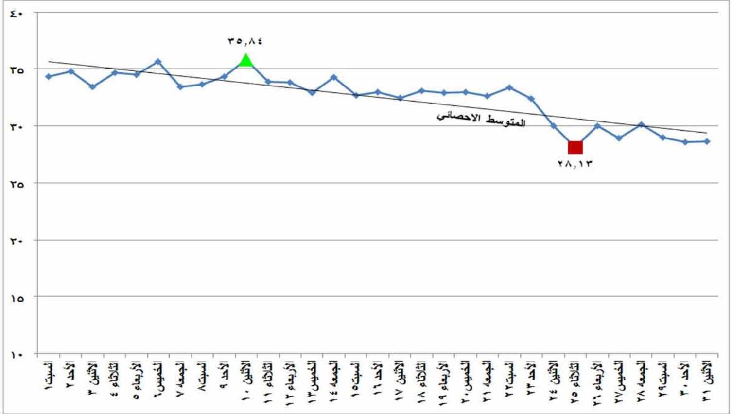
شكل (٢٣) الطاقة الكهربائية المنتجة من المصادر المائية خلال شهر أكتوبر ٢٠١٦
