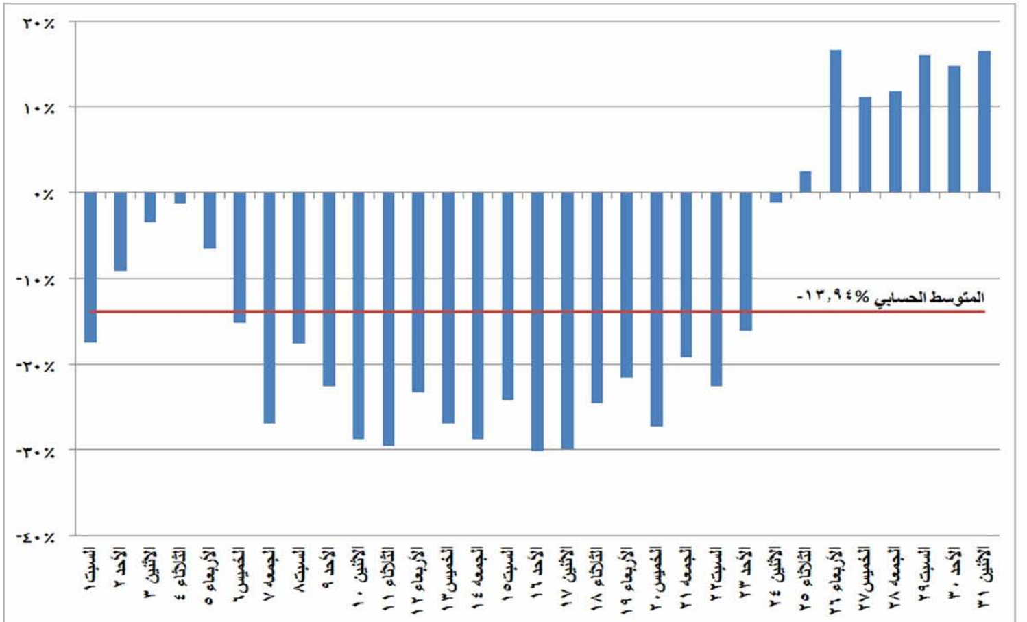
شكل (٢٠) نسب التغير في استخدام المازوت في إنتاج الطاقة الكهربائية خلال شهر أكتوبر ٢٠١٦ مقارنة بالشهر المماثل من العام السابق
