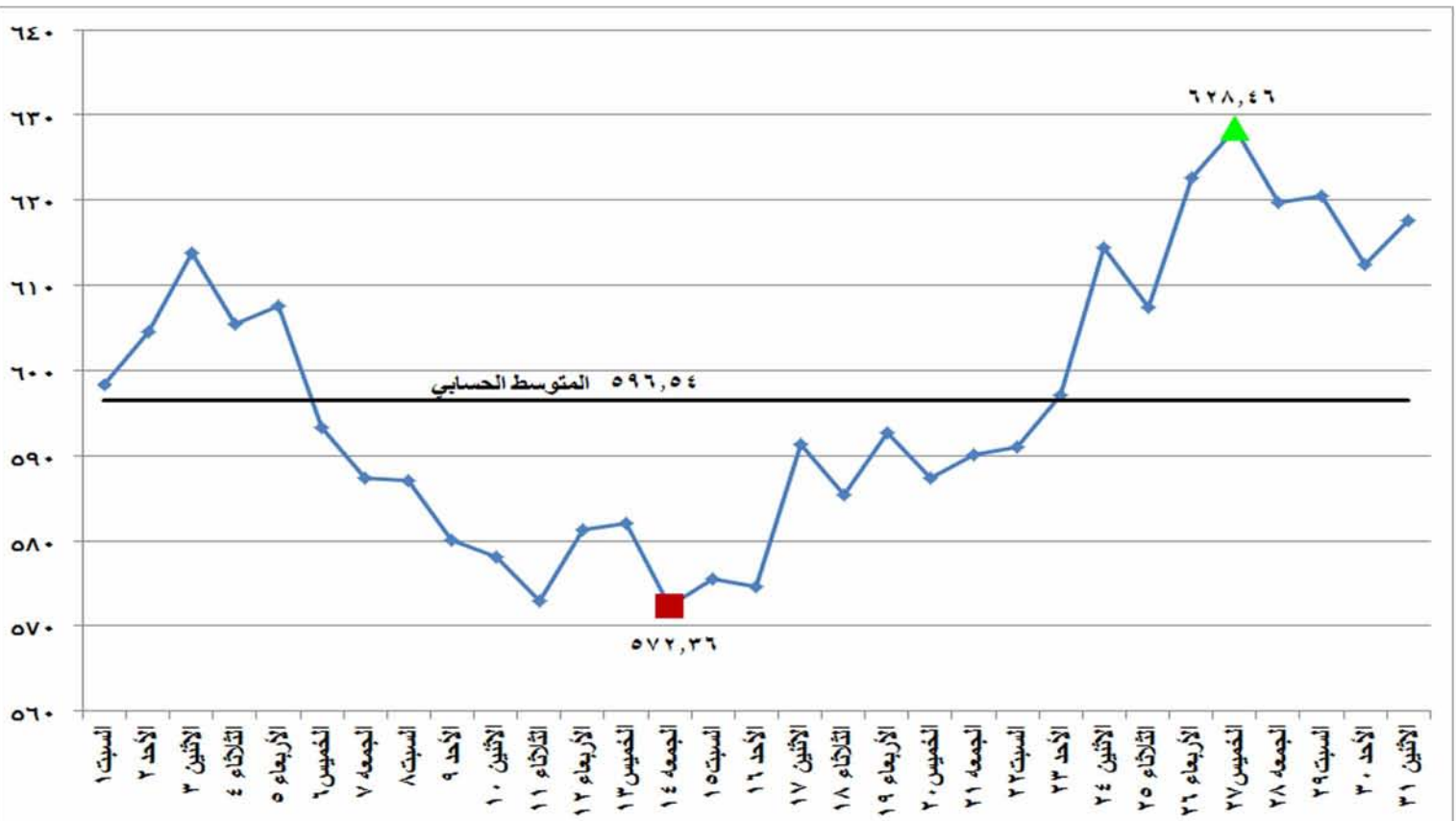
شكل (١٤) معامل انبعاثات غاز ثاني اكسيد الكربون المكافئ على مدى شهر أكتوبر ٢٠١٦
