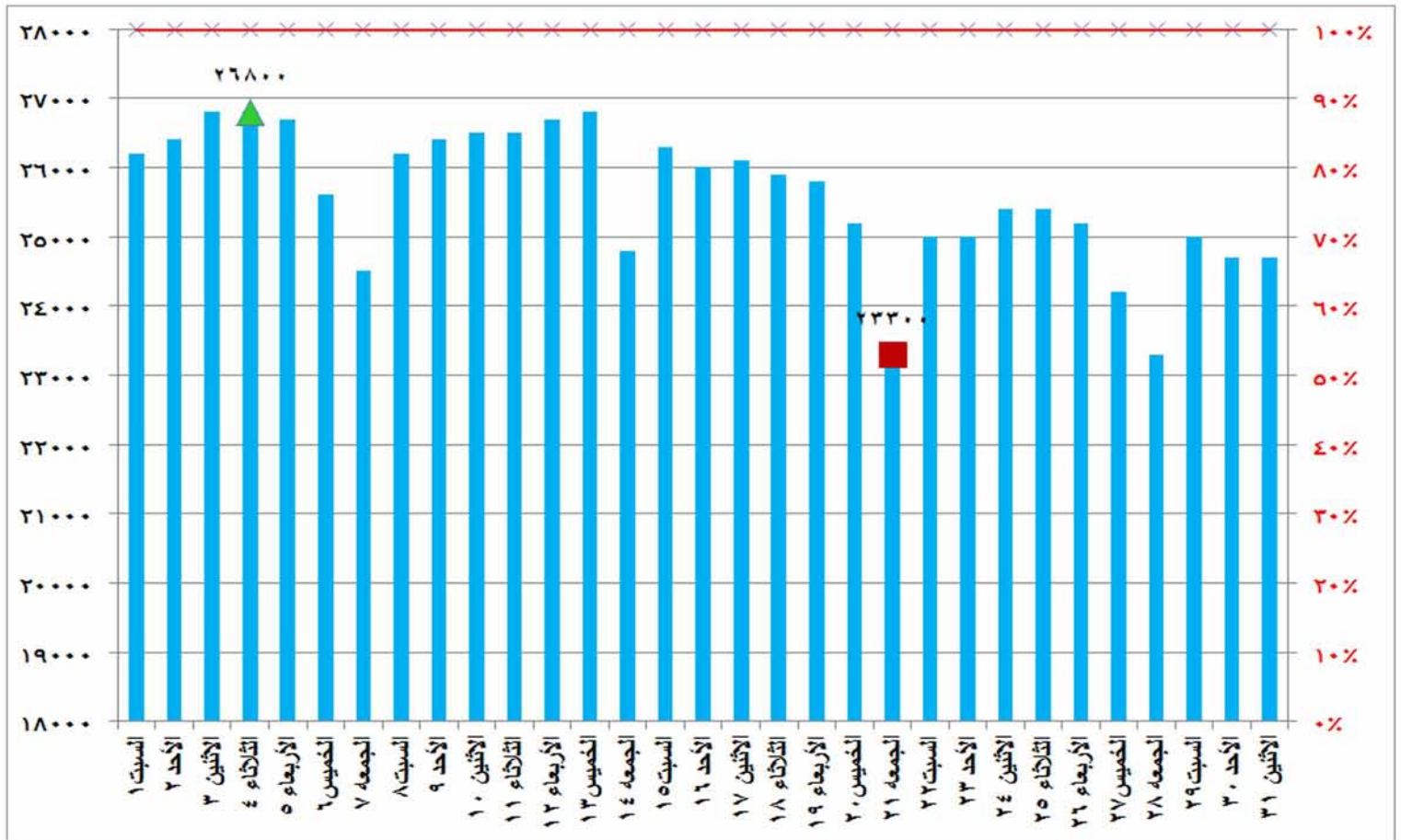
شكل (٥) قدرات الانتاج المتاحة ونسبتها للحمل الأقصى خلال شهر أكتوبر ٢٠١٦
