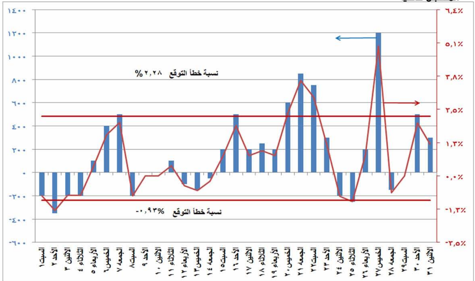
شكل (١٠) الفرق بين الحمل الأقصى المتوقع والمسجل فعليا ونسبة الفرق إلى الحمل المسجل فعليا خلال شهر أكتوبر ٢٠١٦
