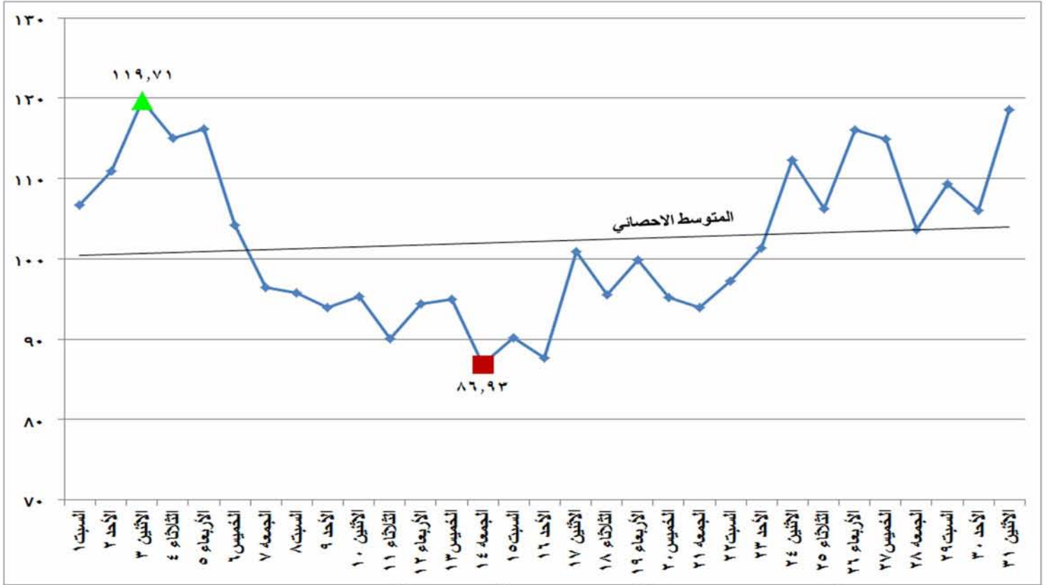
شكل (١٩) الطاقة الكهربائية المنتجة من المازوت خلال شهر أكتوبر ٢٠١٦
