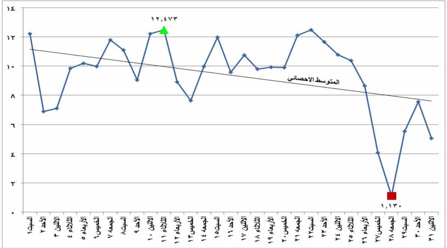
شكل (٢٥) الطاقة الكهربائية المنتجة من الرياح والشمس خلال شهر أكتوبر ٢٠١٦
