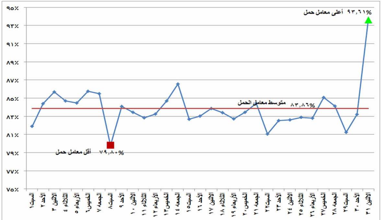
شكل (١٢) إجمالي معامل الحمل لوحدات الانتاج خلال شهر أكتوبر ٢٠١٦
