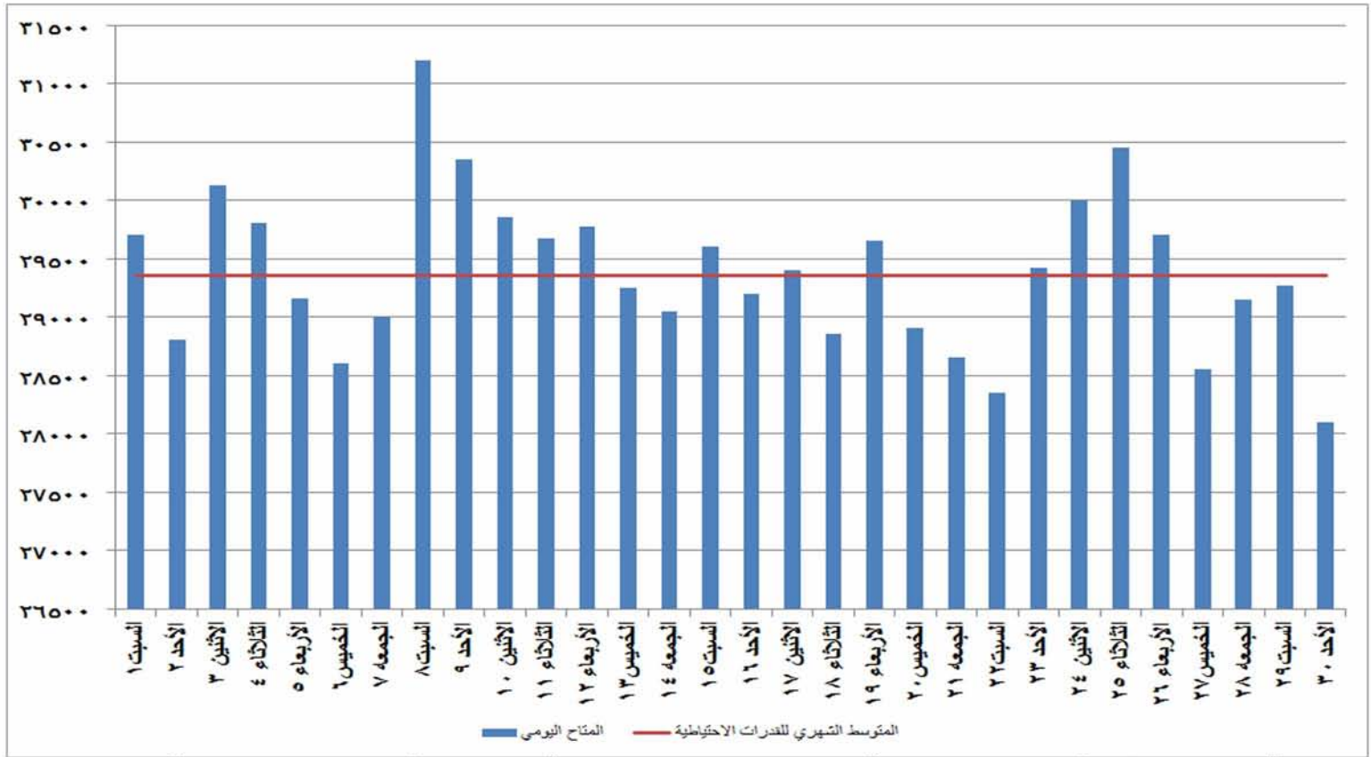
شكل (٢٧) القدرات المتاحة يوميا والمتوسط الشهري للقدرة الاحتياطية خلال شهر أكتوبر ٢٠١٦
