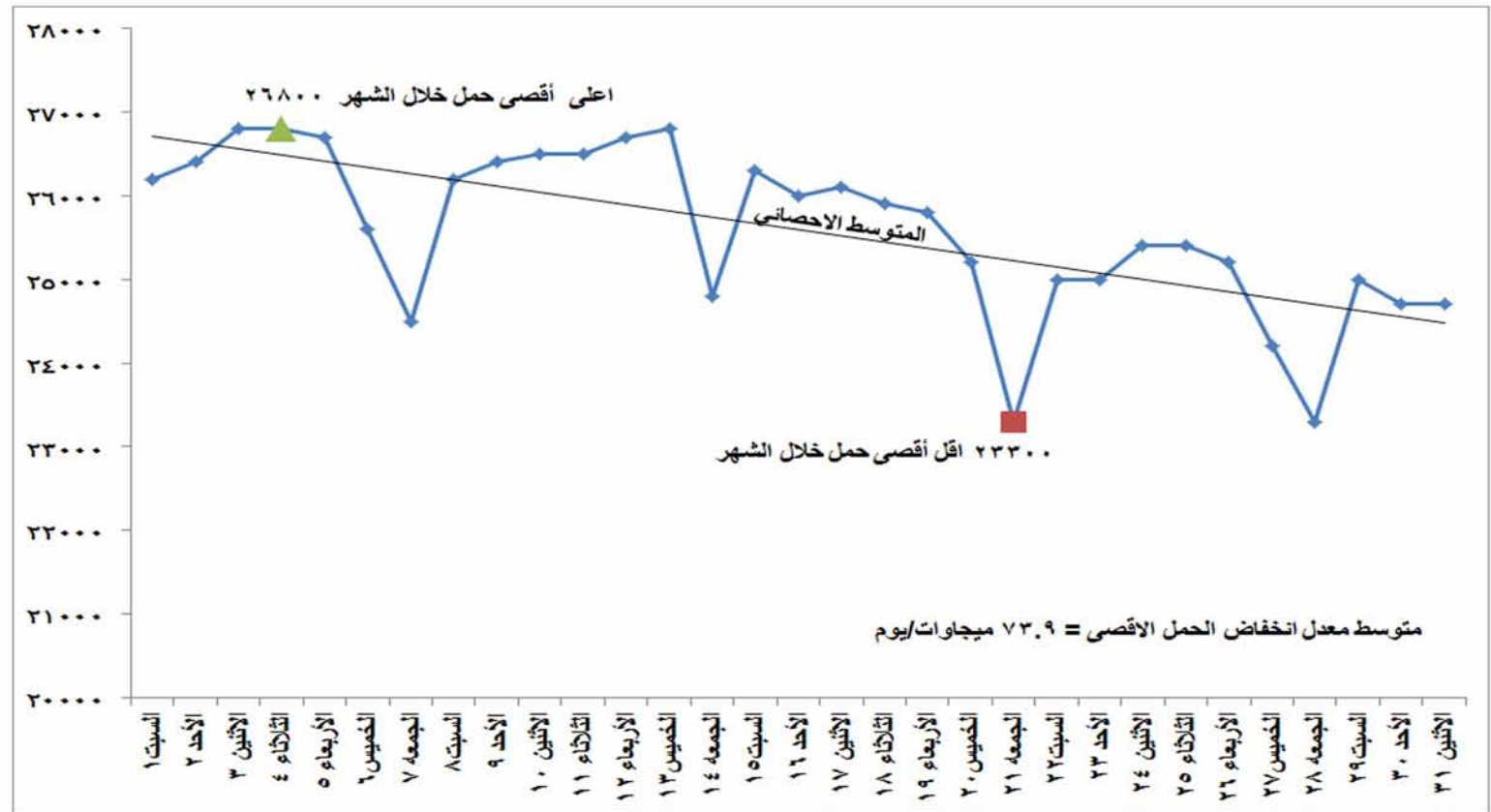
شكل (١) تطور الحمل الاقصى اليومي خلال شهر أكتوبر ٢٠١٦
