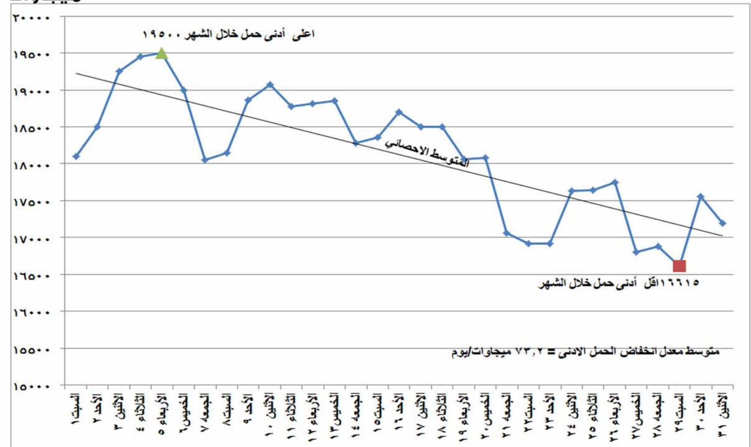
شكل (٢) تطور الحمل الادنى اليومي خلال شهر أكتوبر ٢٠١٦
