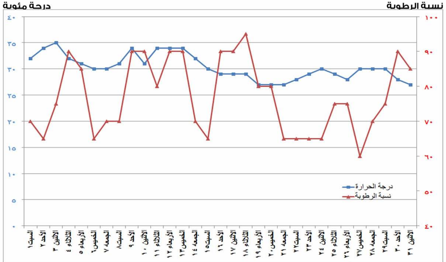
شكل (١١) التغيير في درجة الحرارة والرطوبة النسبية خلال شهر أكتوبر ٢٠١٦
